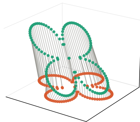
Lemniscate
